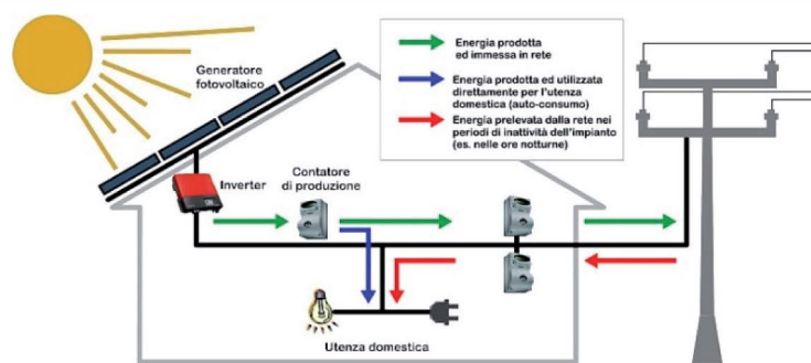
Schema di impianto fotovoltaico domestico
